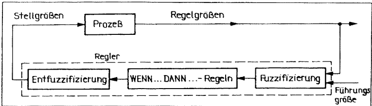
Abbildung 3: Fuzzy-Regelung
